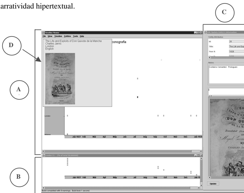
Fig. 1. ItLv mostrando parte de la iconografía del Quixote en cuatro niveles; a) una vista general, b) una ventanilla detallando la categoría, c) una ventanilla con el detalle de cada elemento, y d) una ventanilla indicando ciertos atributos de la información (el usuario puede escoger los atributos que desee).
